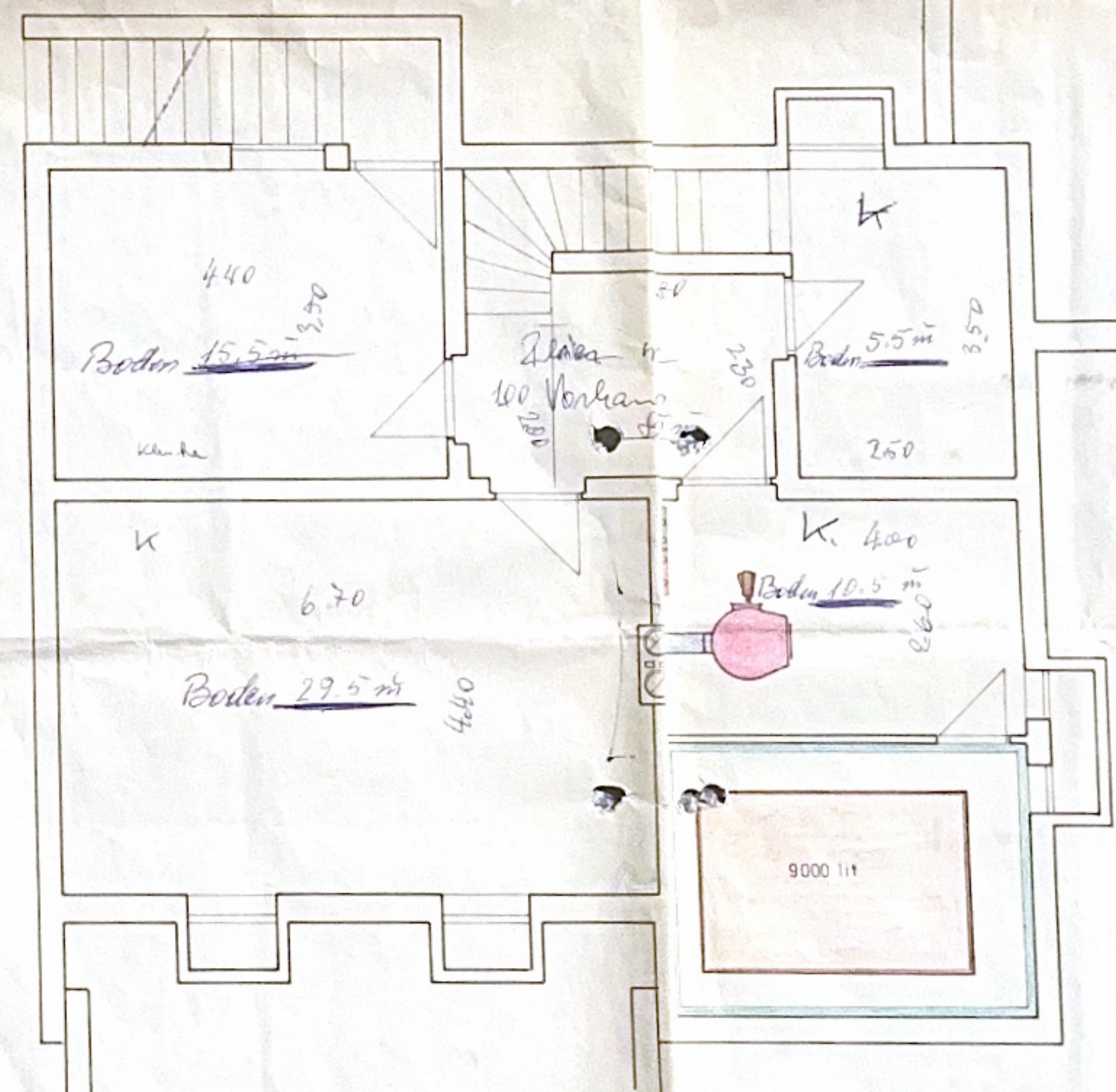
KELLER
