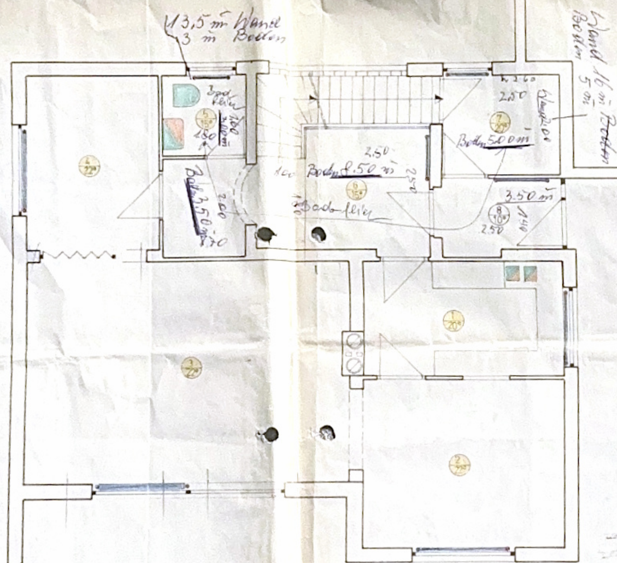
ERDGESCHOSS
